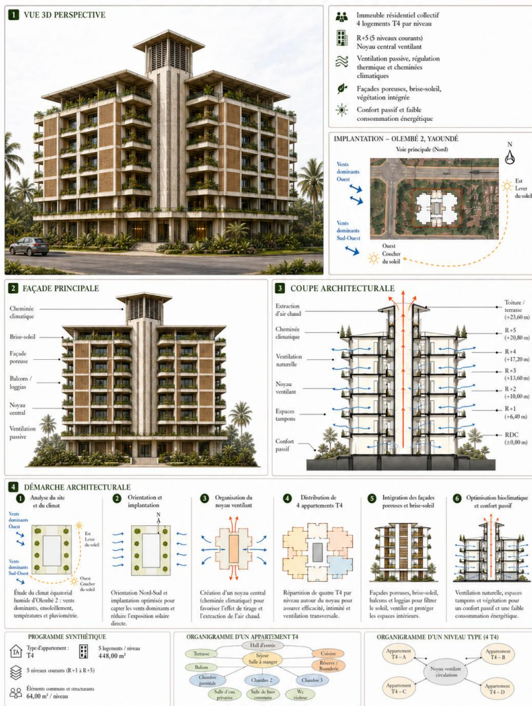
Figure 3.xx : Variante retenue – Termitière climatique
